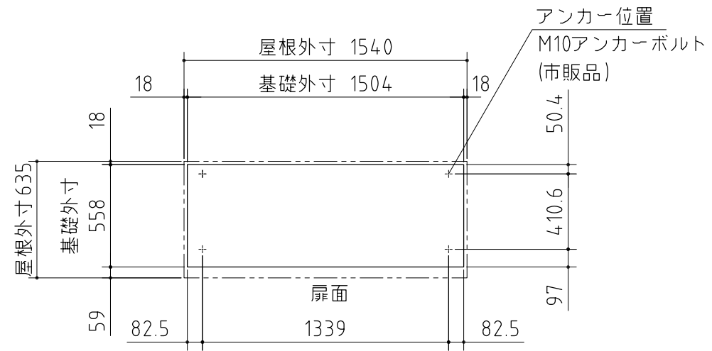
ベタ基礎図
